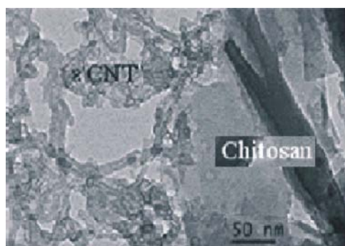
Fig. 8: TEM OF MWCNT-CHITOSAN
